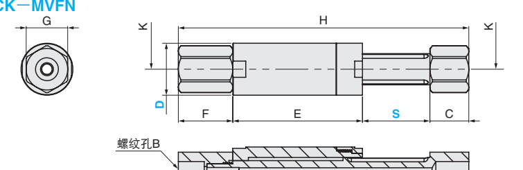
K—K视图
