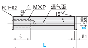
MSTP (带拉拔螺纹精密型)
