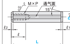
MSTH (带拉拔螺纹h7型)
