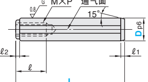
MST (带拉拔螺纹p6型)
