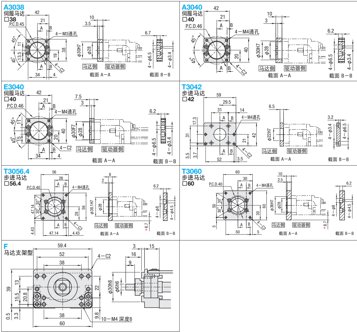
■马达附件尺寸图
