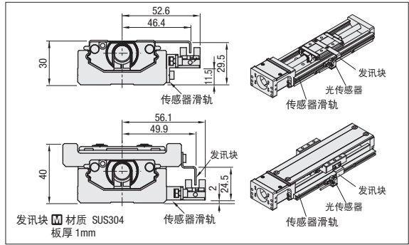
■光传感器型安装图 SUNX制造/OMRON制造
