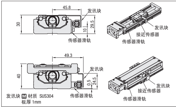
■接近传感器型安装图 SUNX制造
