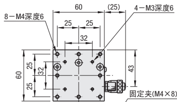
ZLPGS60(千分尺旋钮 螺距0.5)
