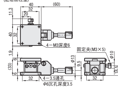
ZLTG40 (进给丝杠型)
