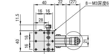
ZLPGS40(千分尺旋钮 螺距0.5)
