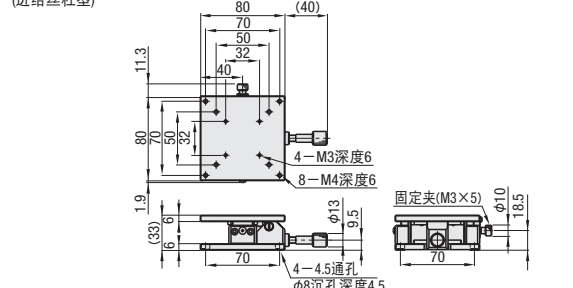
ZLTG80 (进给丝杠型)
