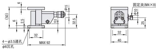
ZLPGS60(千分尺旋钮 螺距0.5)
