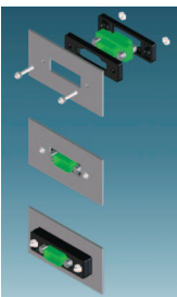
※组装示意图
