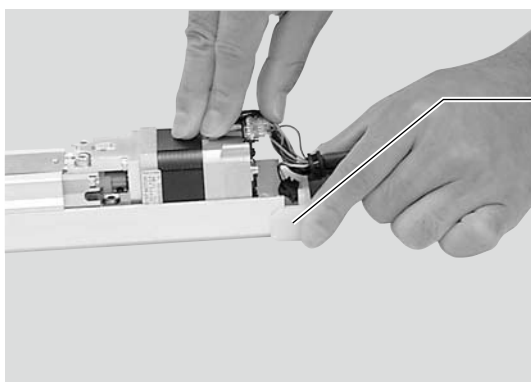
马达盖 2
