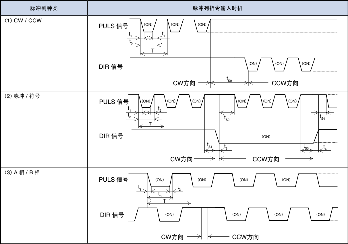
脉冲列指令输入的时机时间
