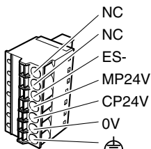
电源连接器
