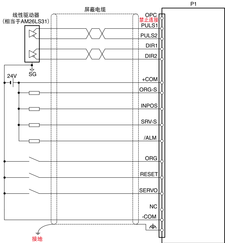
连接示例
