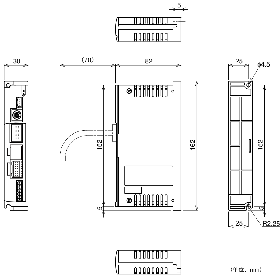
外观尺寸图
