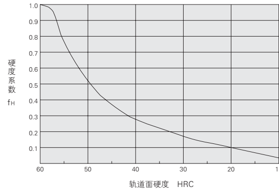
图一1. 硬度系数
